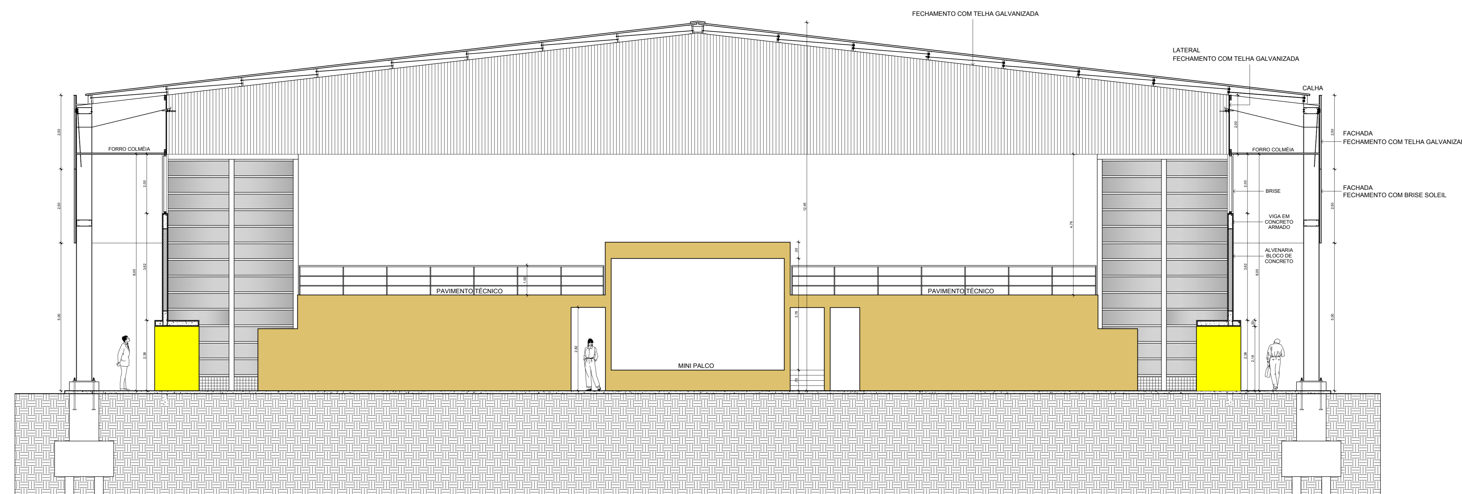
CORTE BB - GINÁSIO POLIESPORTIVO Escala: 1/75
