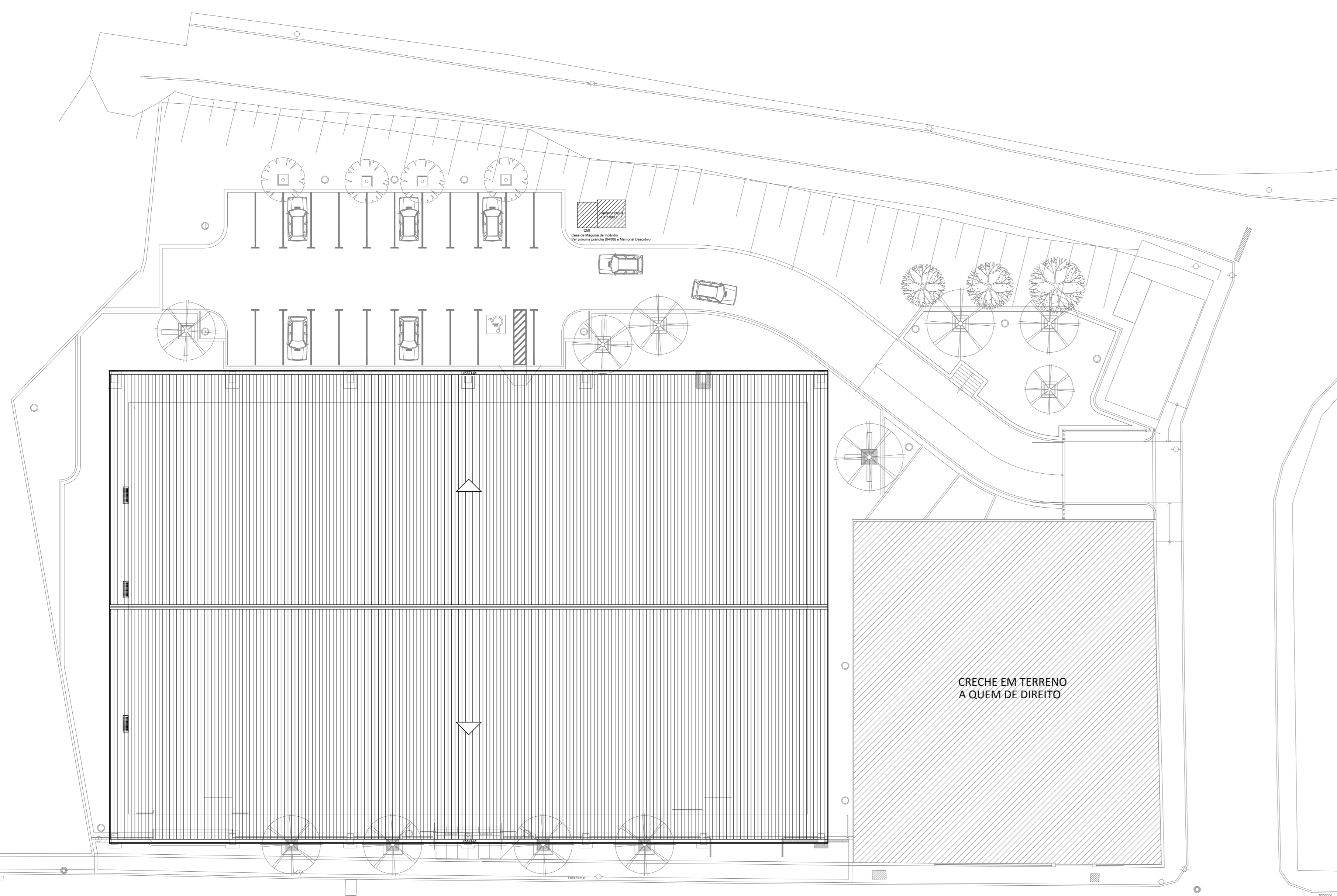
SITUAÇÃO / IMPLANTAÇÃO - GINÁSIO POLIESPORTIVO Escala: 1/250
