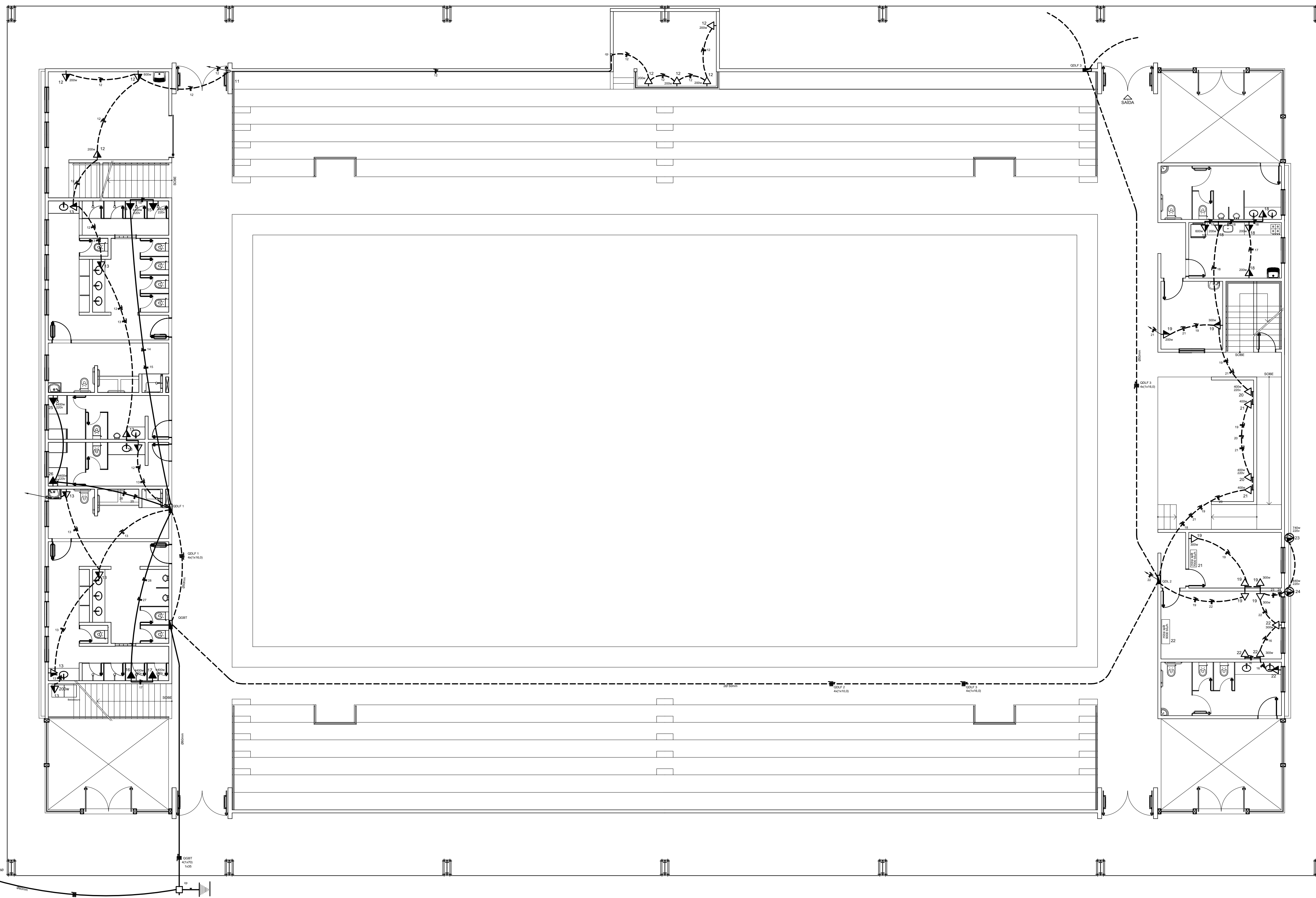
PLANTA BAIXA - TÉRREO - GINÁSIO POLIESPORTIVO Escala: 1 / 100 TOMADAS
