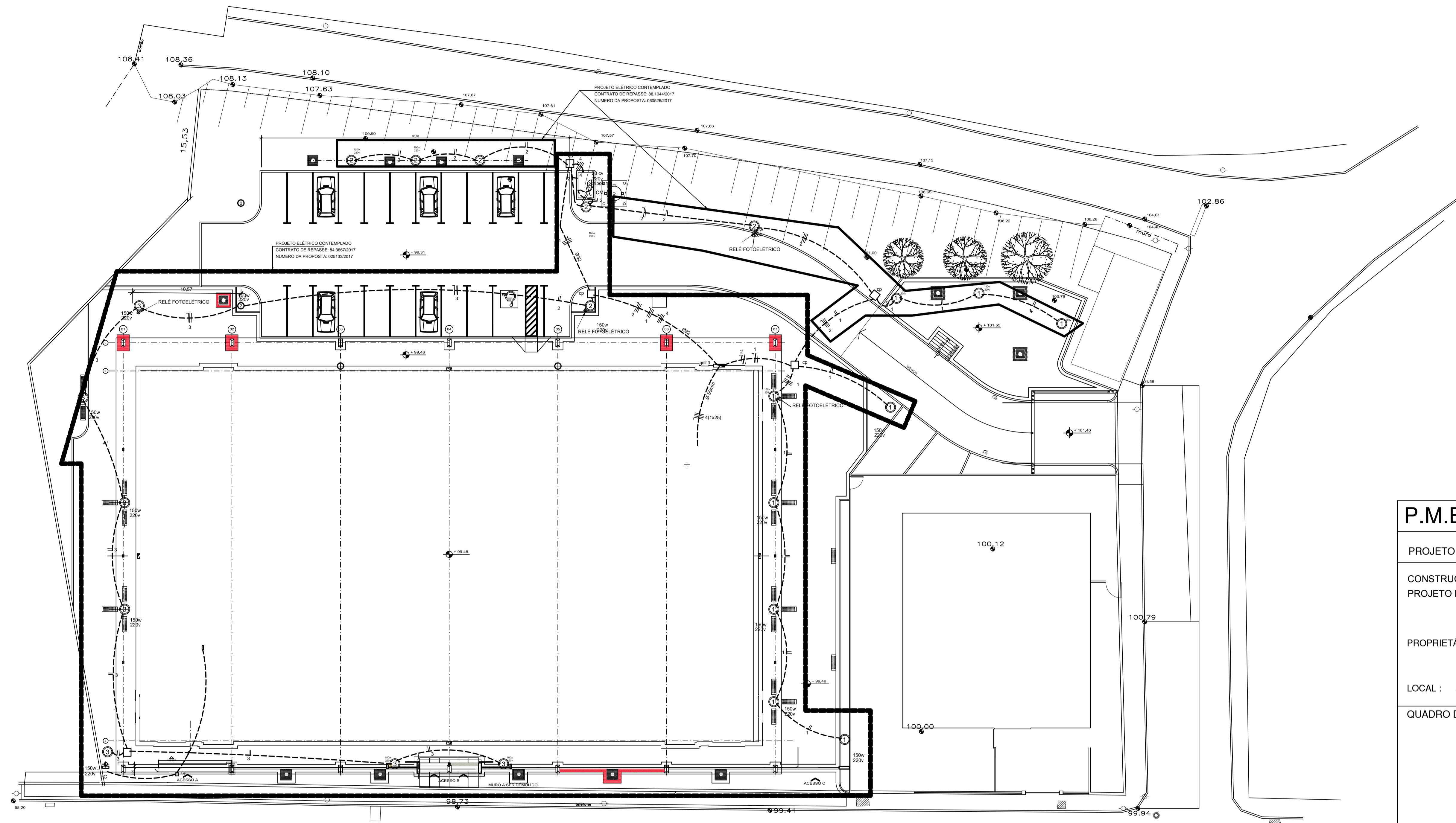
PLANTA BAIXA - SITUAÇÃO - GINÁSIO POLIESPORTIVO ILUMINAÇÃO/FORÇA Escala Gráfica: 0 1m 5m 10m
