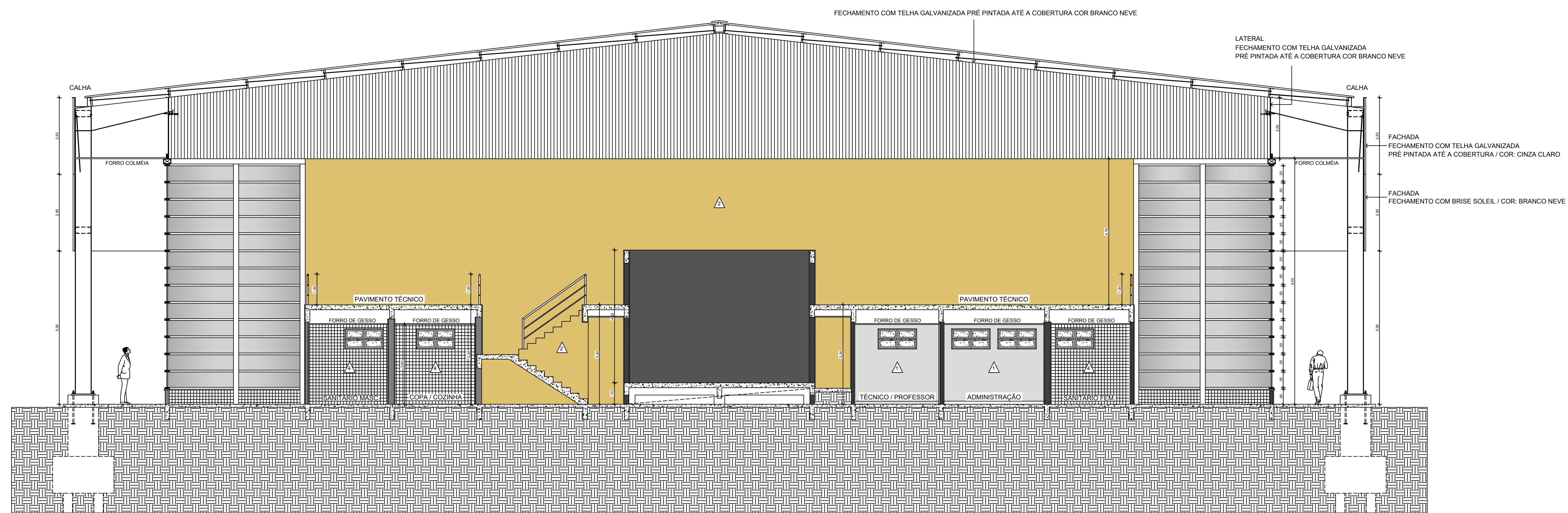
02 CORTE FF - GINÁSIO POLIESPORTIVO Escala: 1/75
