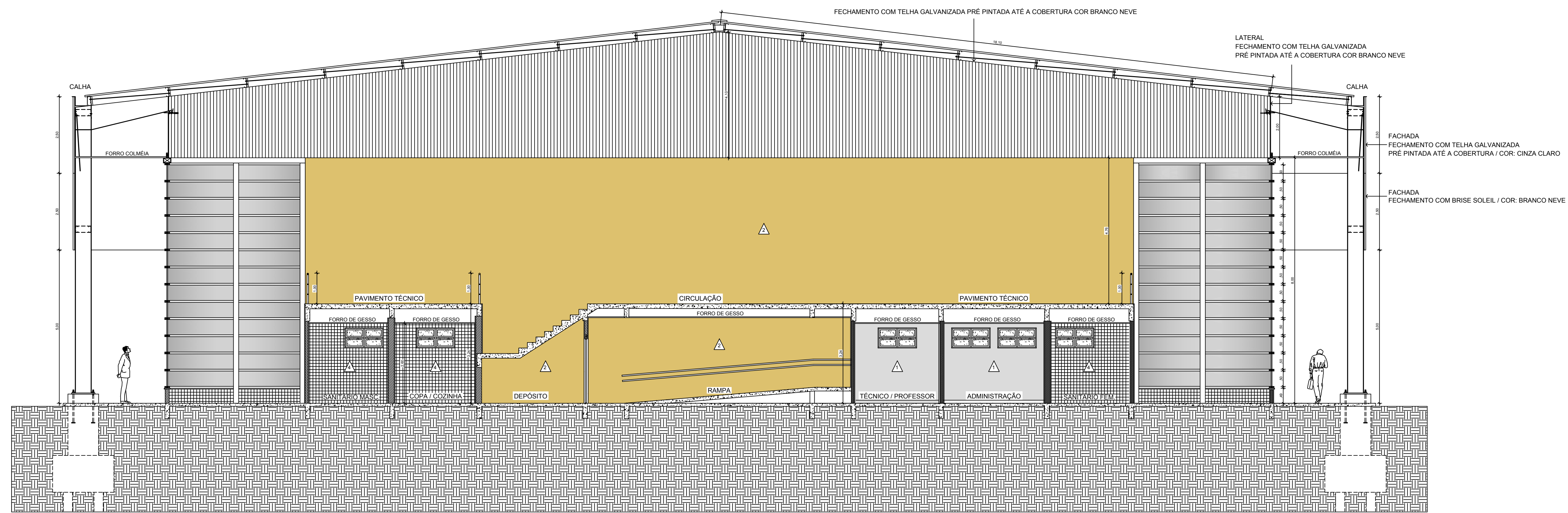
01 CORTE EE - GINÁSIO POLIESPORTIVO Escala: 1/75
