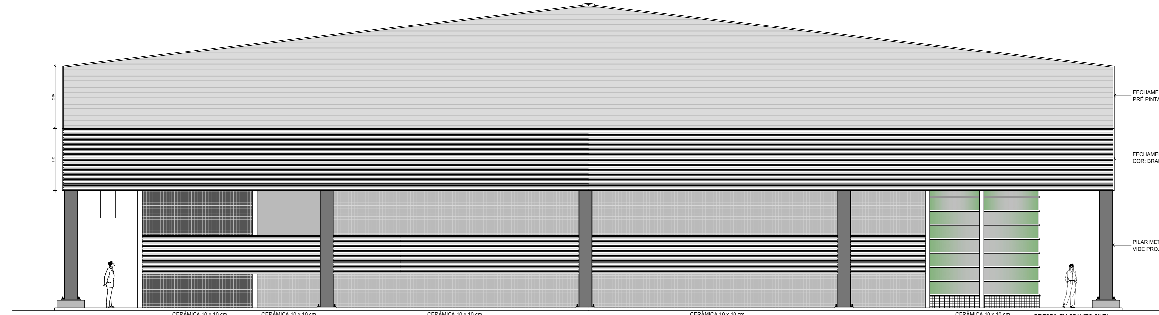
04 FACHADA 04 - LATERAL - GINÁSIO POLIESPORTIVO Escala: 1/75 Escala Gráfica: 0 1m 5m 10m
