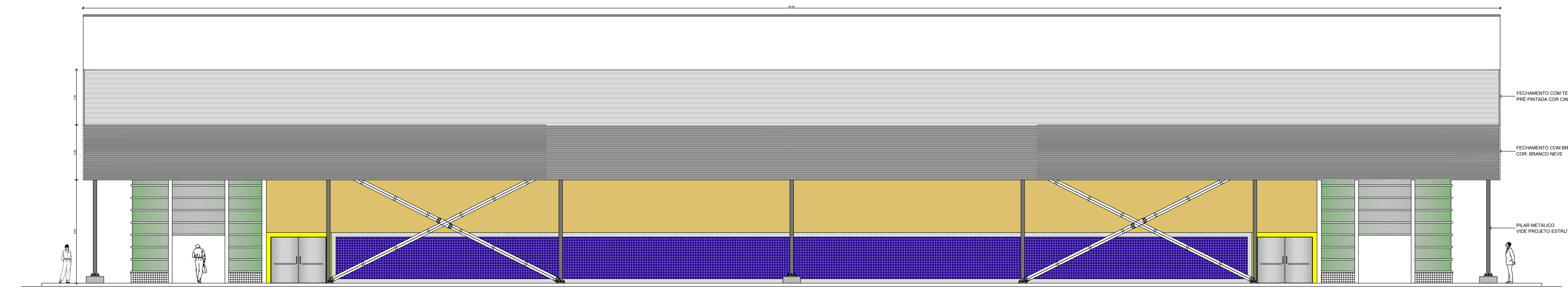
01 FACHADA 01 - FRONTAL - GINÁSIO POLIESPORTIVO Escala: 1/75 0 1m 5m 10m
