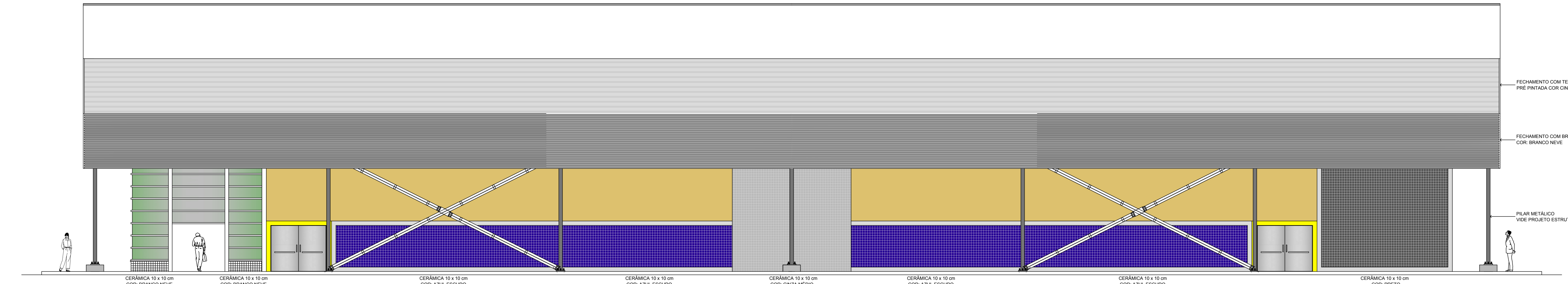
02 FACHADA 02 - FUNDOS - GINÁSIO POLIESPORTIVO Escala: 1/75 0 1m 5m 10m
