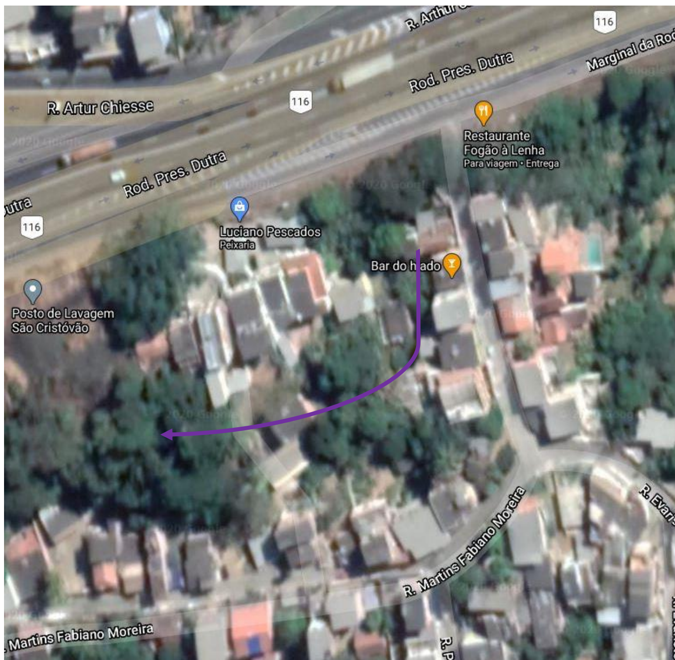
Figura 1: Traçado da Rede Coletora
