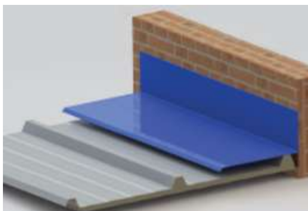
Imagem 7 – Rufo lateral.
