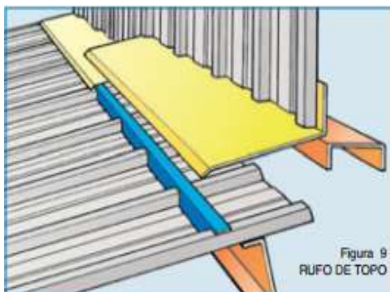
Imagem 12 – Rufo de topo. Fonte: Belmetal.
