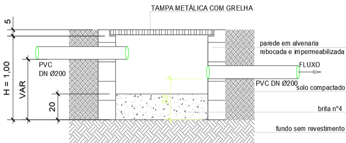
Imagem 14 – Caixa de areia.
