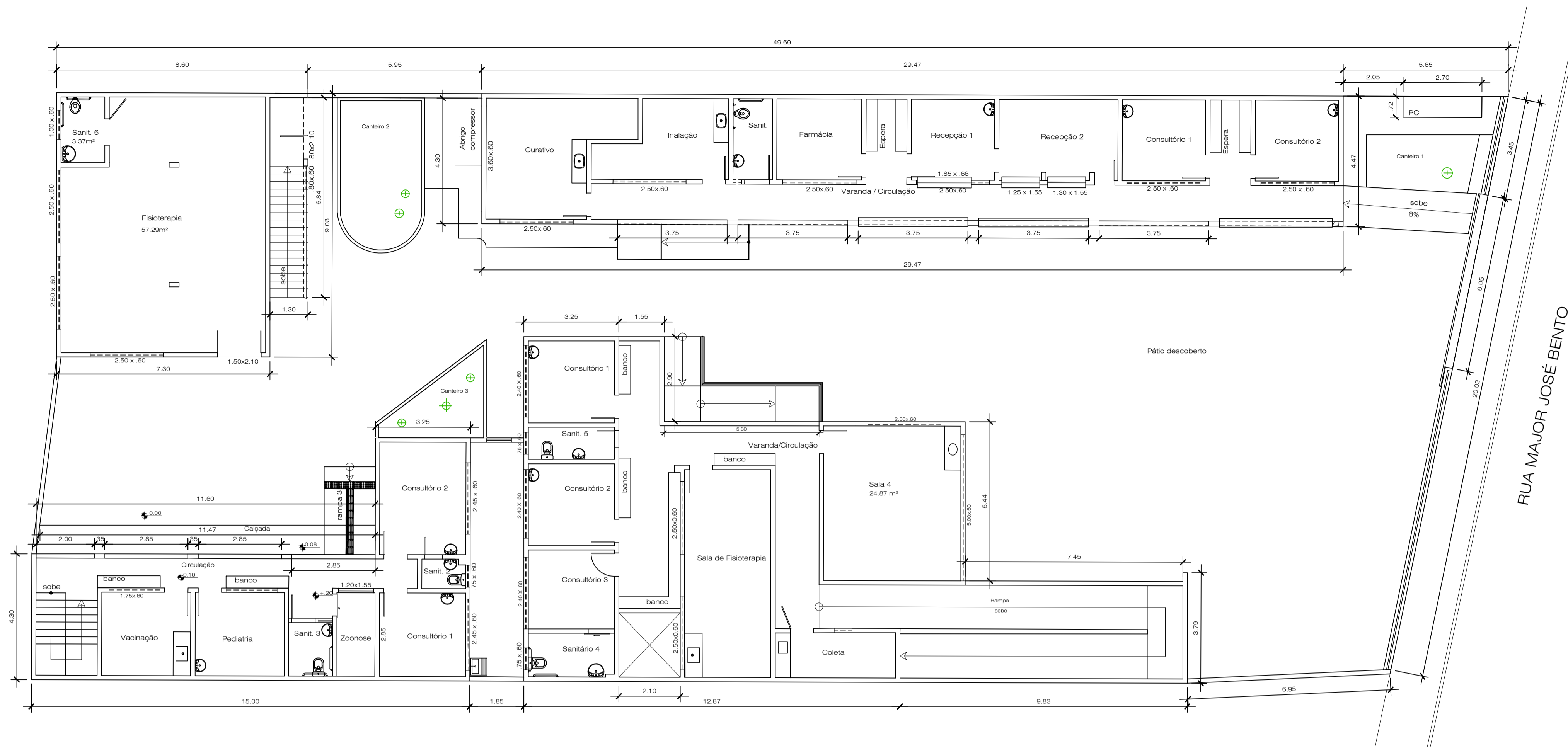
1 PLANTA-BAIXA - TÉRREO Escala 1:100
