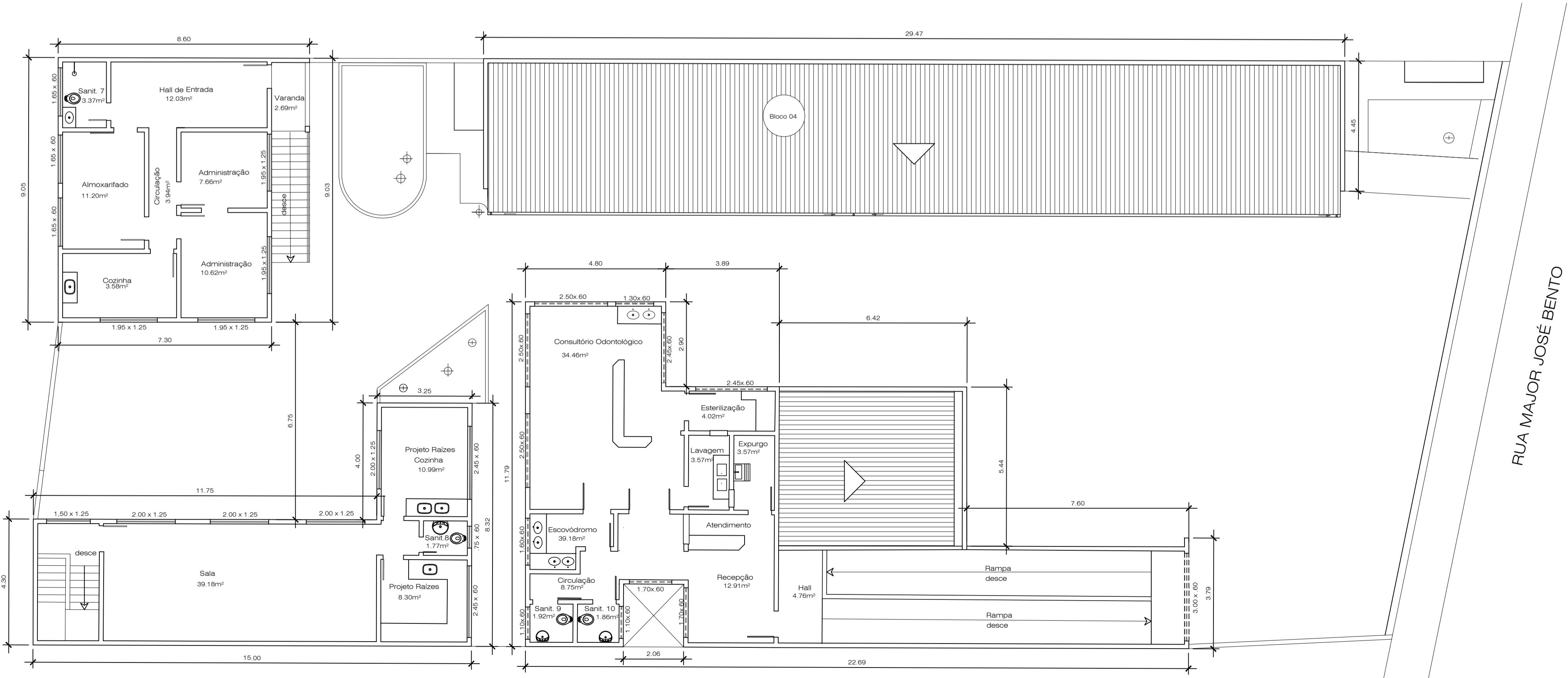
2 PLANTA-BAIXA - 1º PAVIMENTO Escala 1:100
