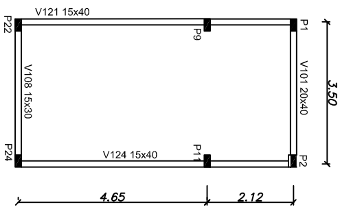
PLANTA FORMAS NIVEL +6,00 esc 1:125
