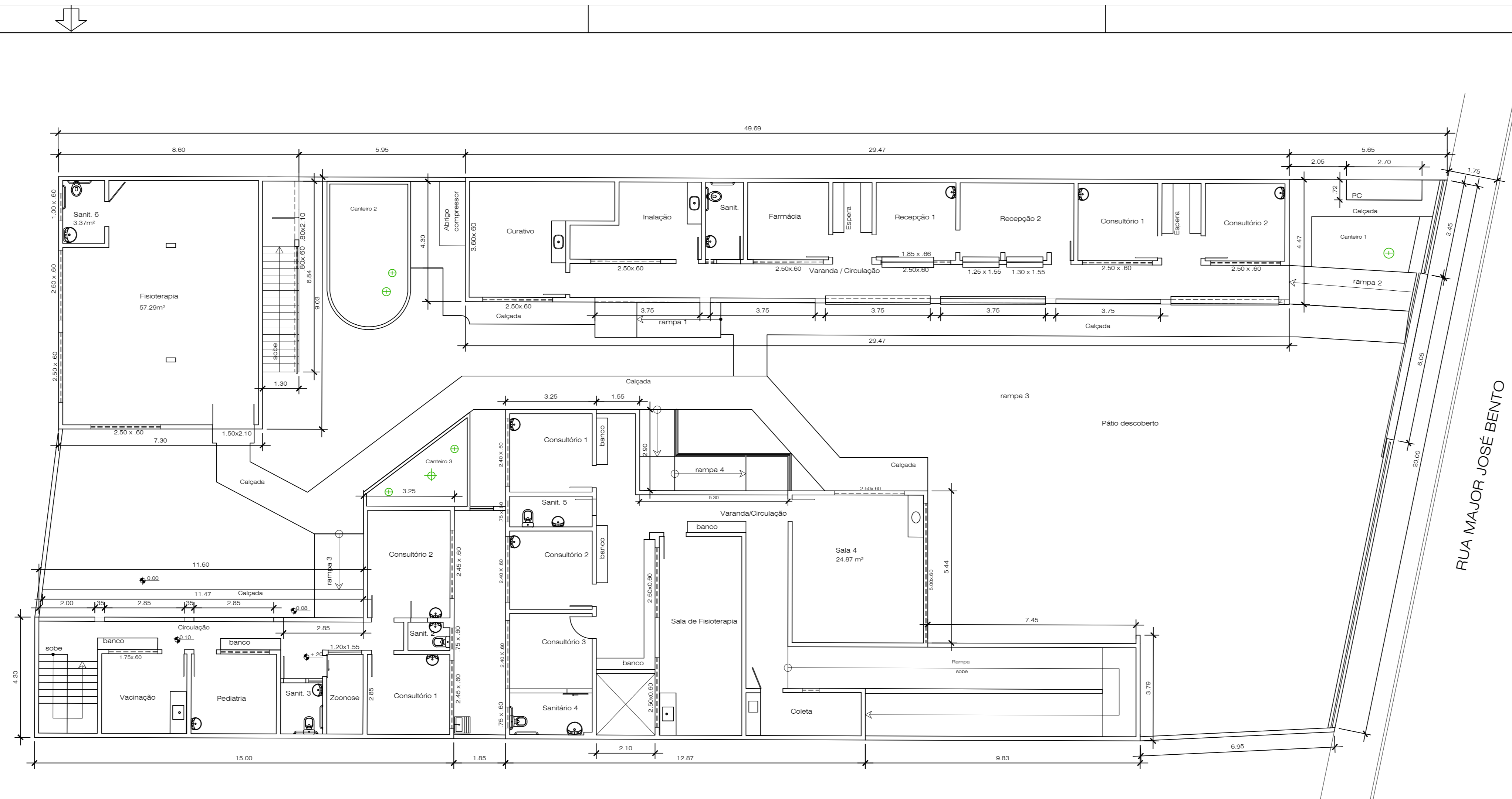
1 PLANTA-BAIXA - TÉRREO Escala 1:100
