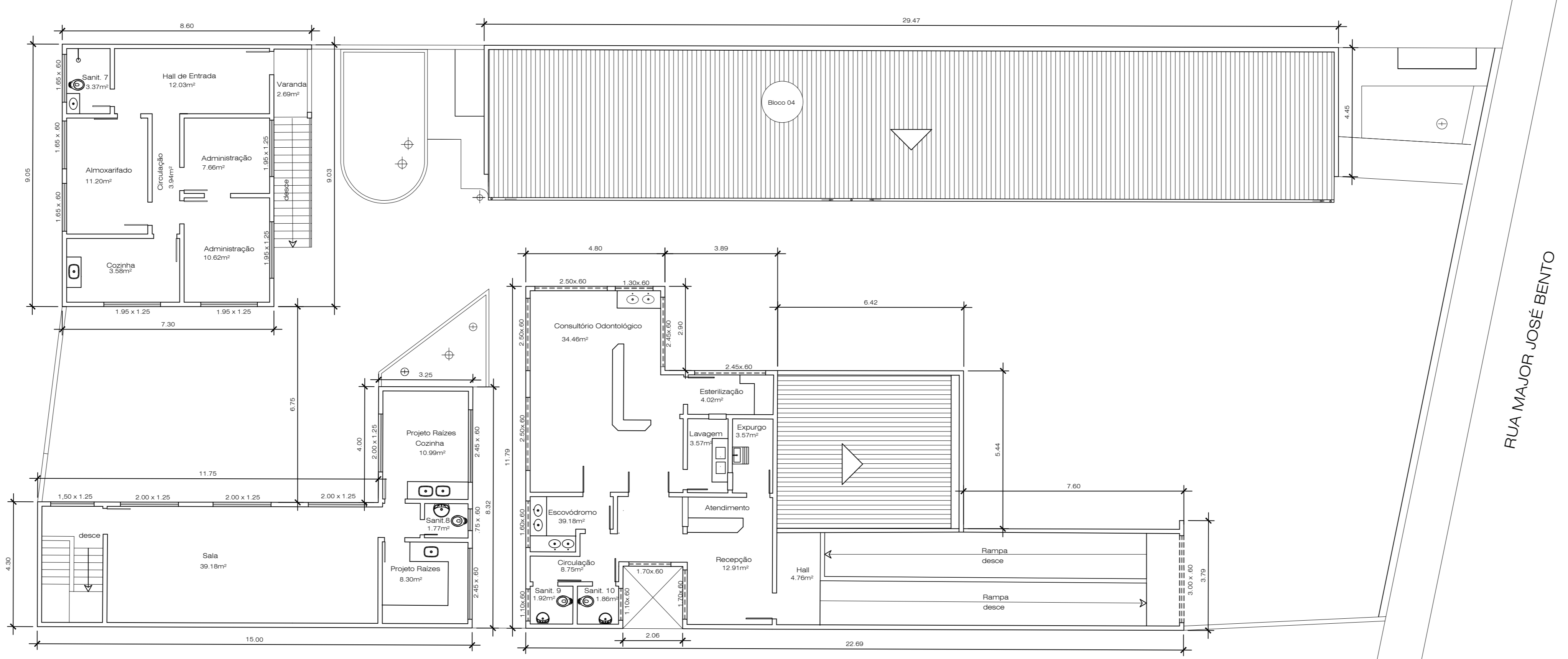
2 PLANTA-BAIXA - 1º PAVIMENTO Escala 1:100
