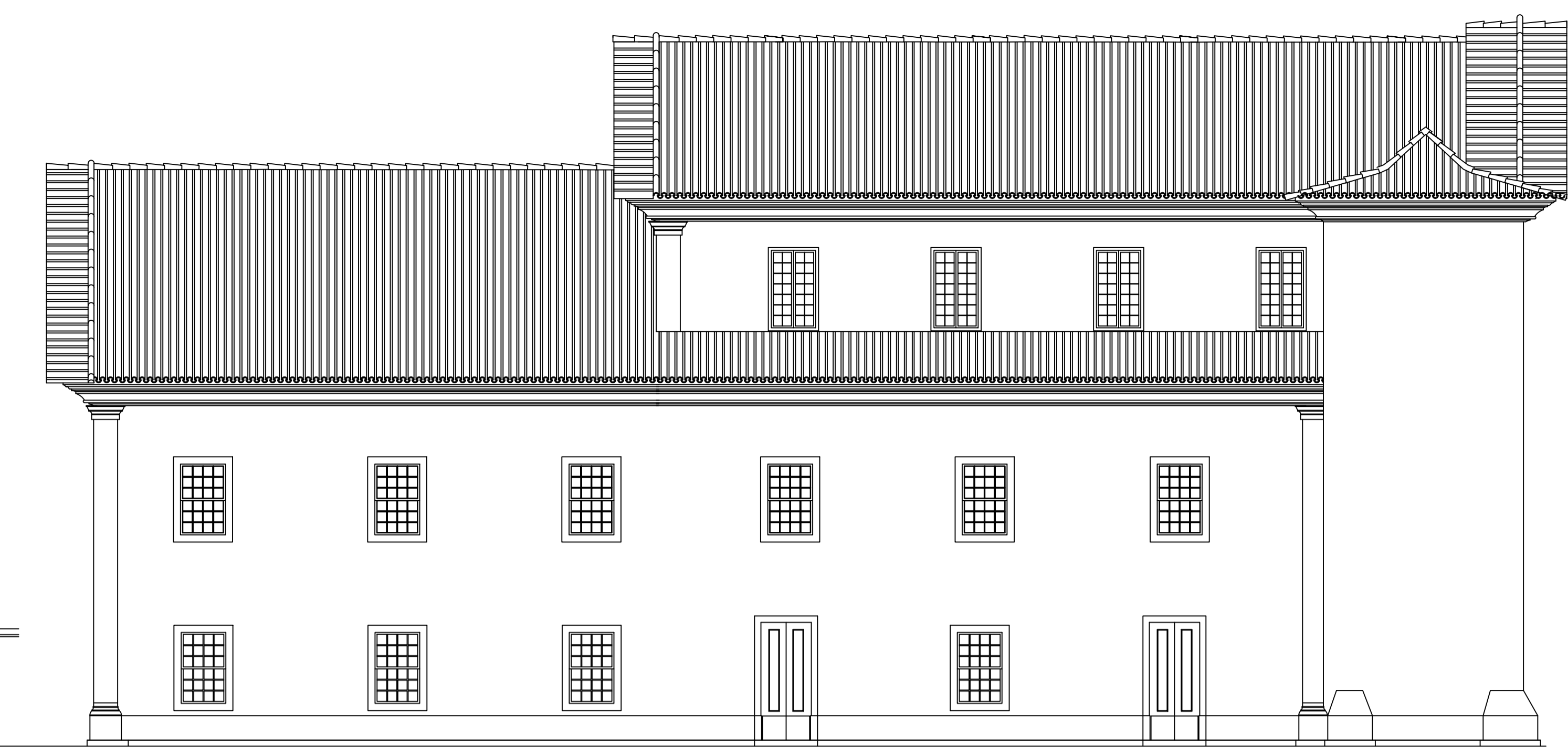
FACHADA LATERAL DIREITA Escala 1:100
