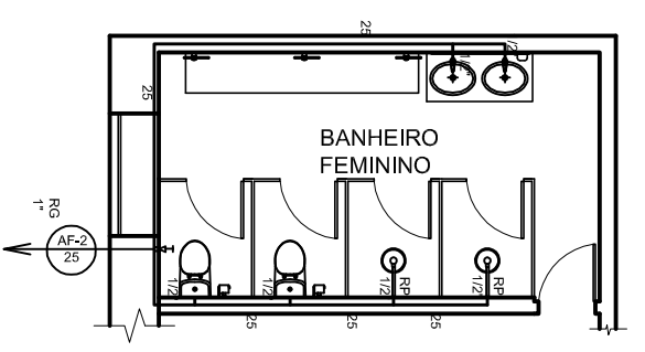
INSTALAÇÃO HIDRAULICA esc 1:100
