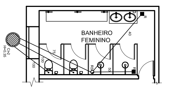
INSTALAÇÃO DE ESGOTO esc 1:100
