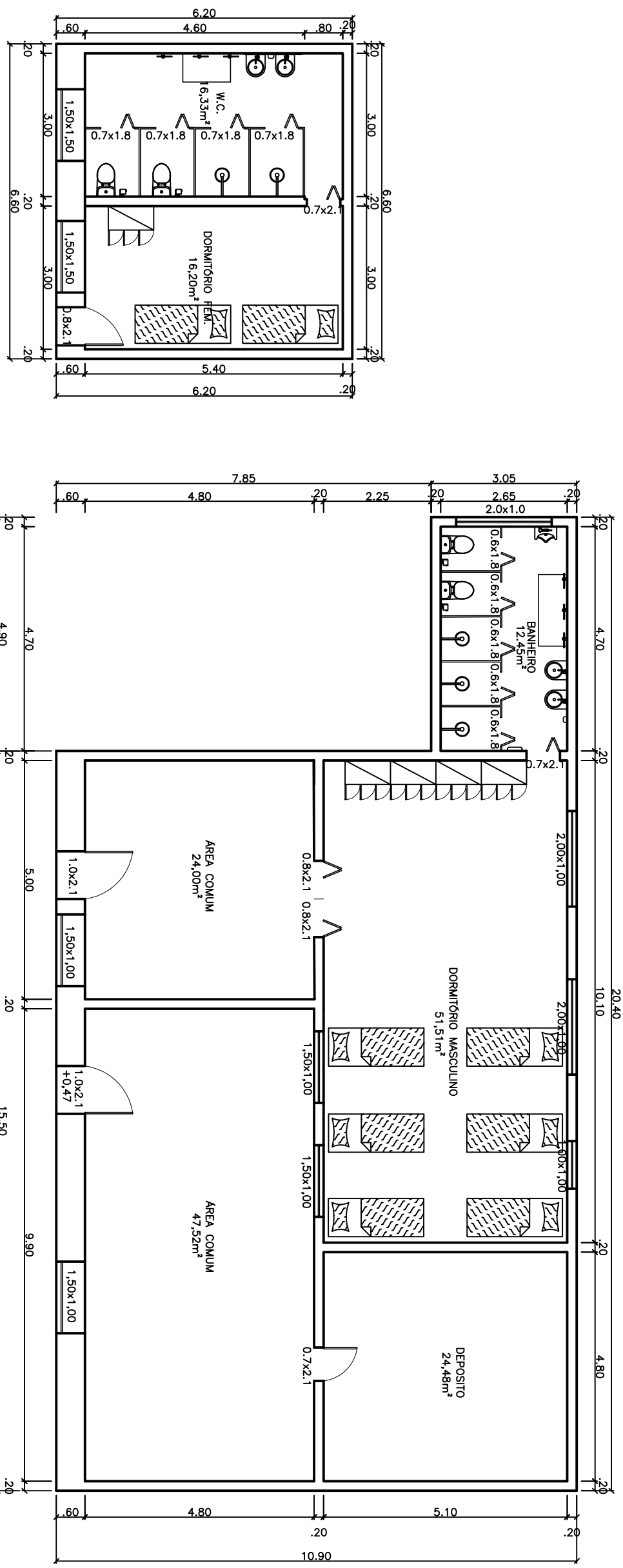
PLANTA BAIXA PROPOSTA esc 1:100
