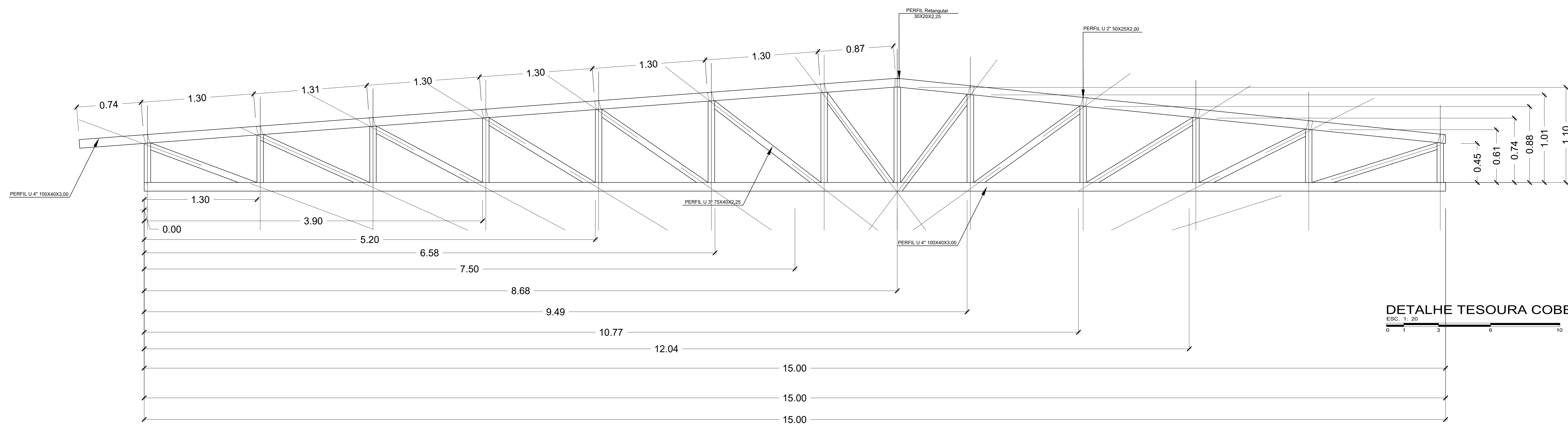
DETALHE TESOURA COBERTURA 3 ESC. 1: 20
