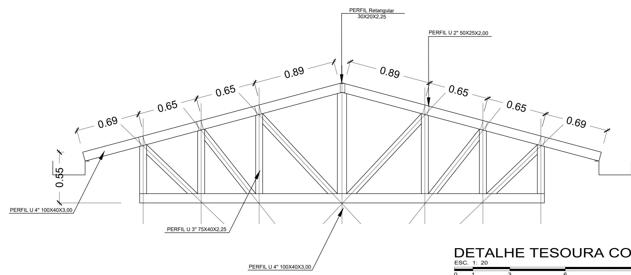
DETALHE TESOURA COBERTURA 2 ESC. 1: 20
