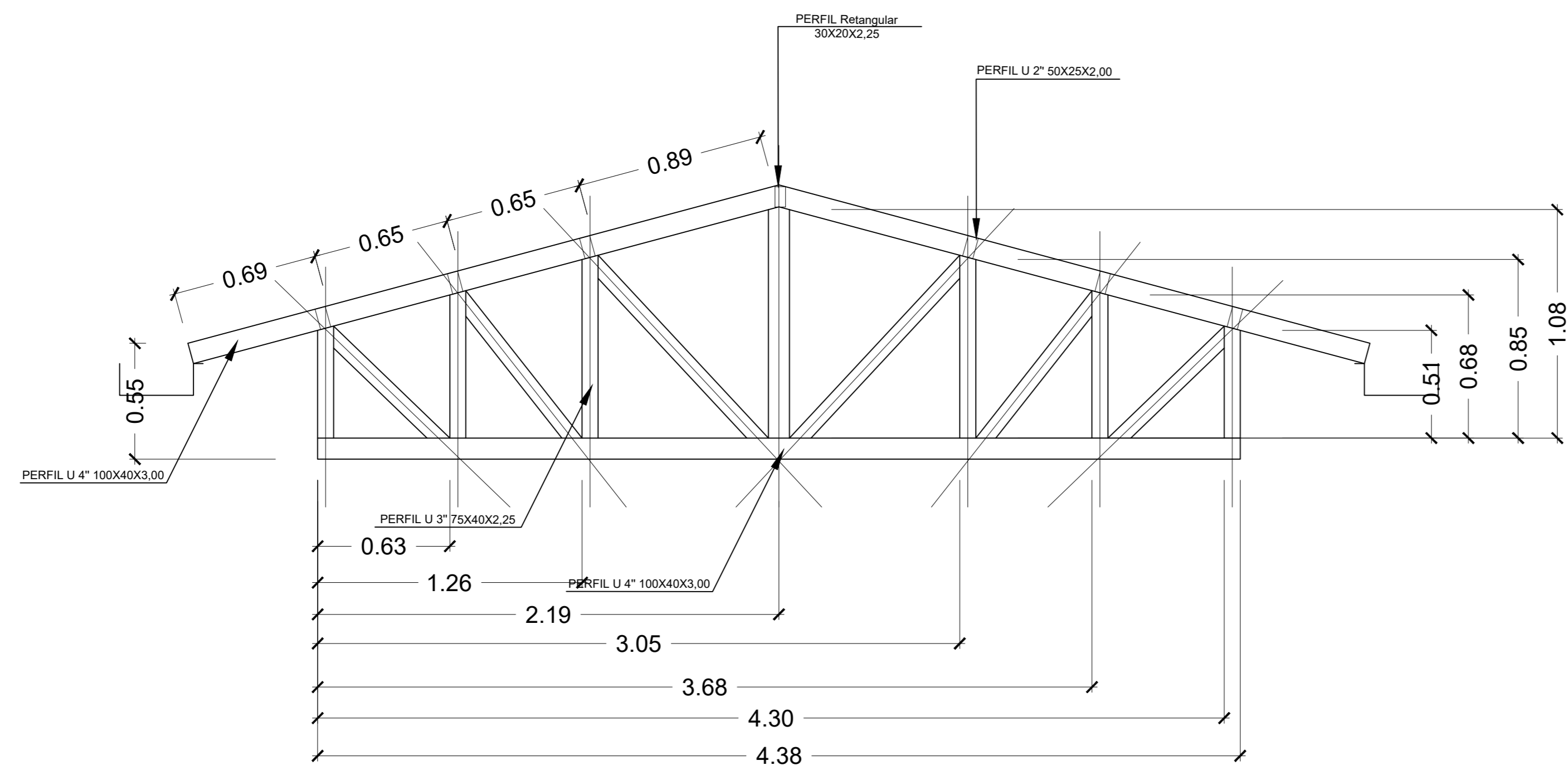
DETALHE TESOURA COBERTURA 2 ESC. 1: 20
