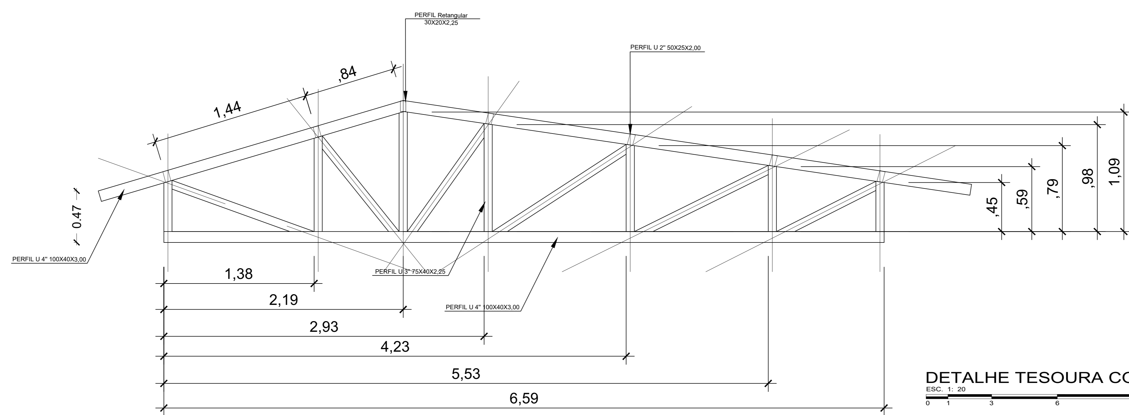
DETALHE TESOURA COBERTURA 2 ESC. 1: 20
