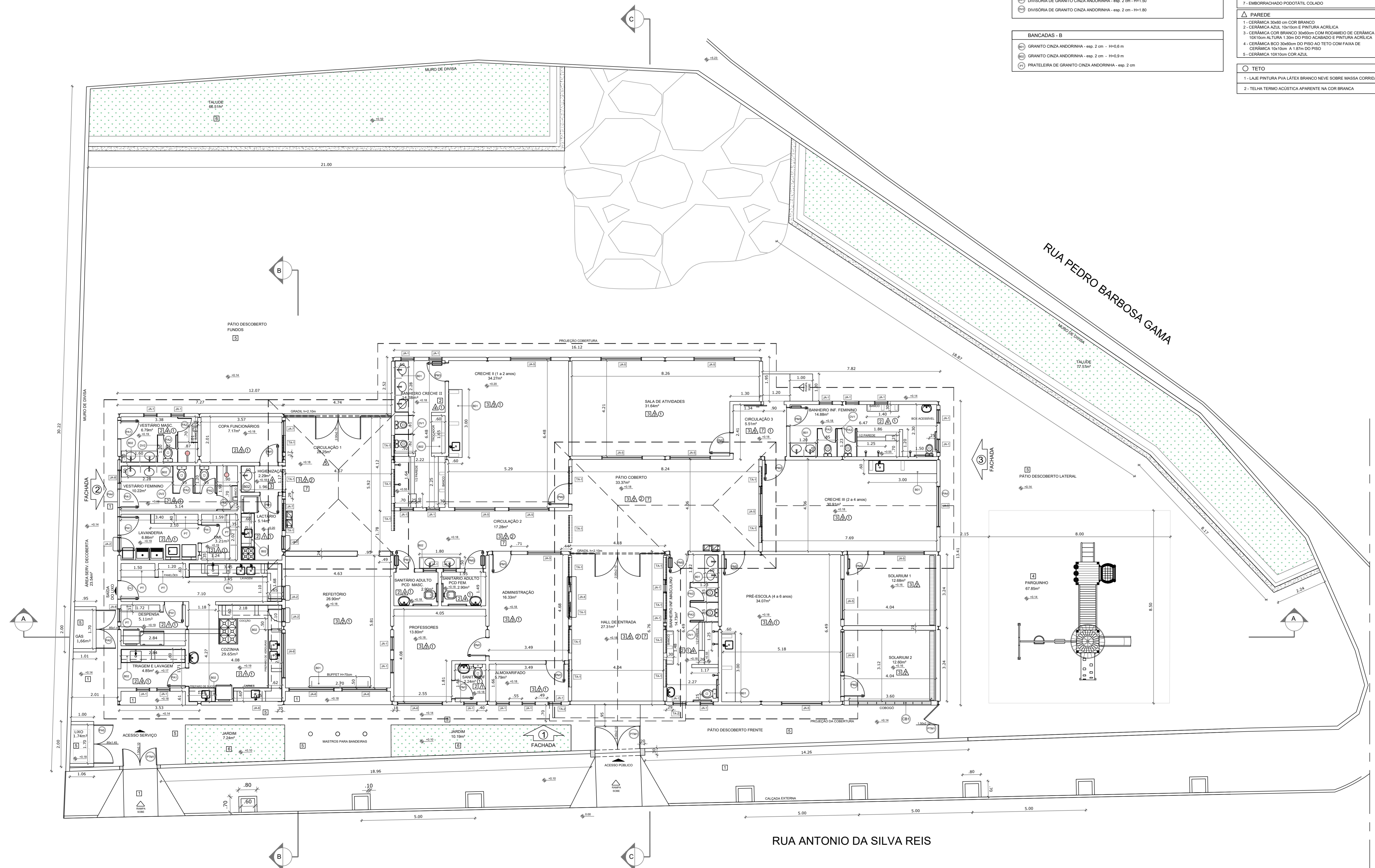
PLANTA-BAIXA esc. 1/75
