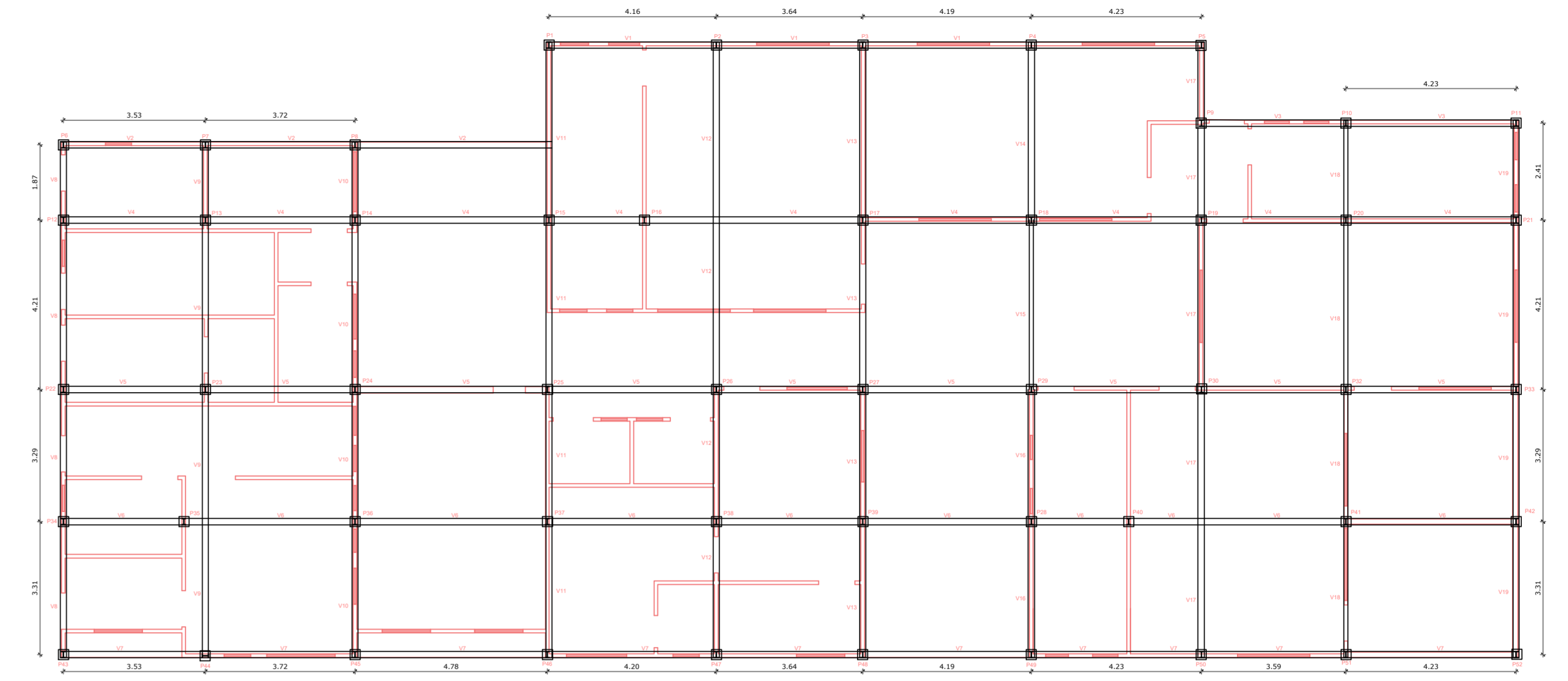
PLANTA -BAIXA - ESTRUTURA METÁLICA EXISTENTE esc. 1/75
