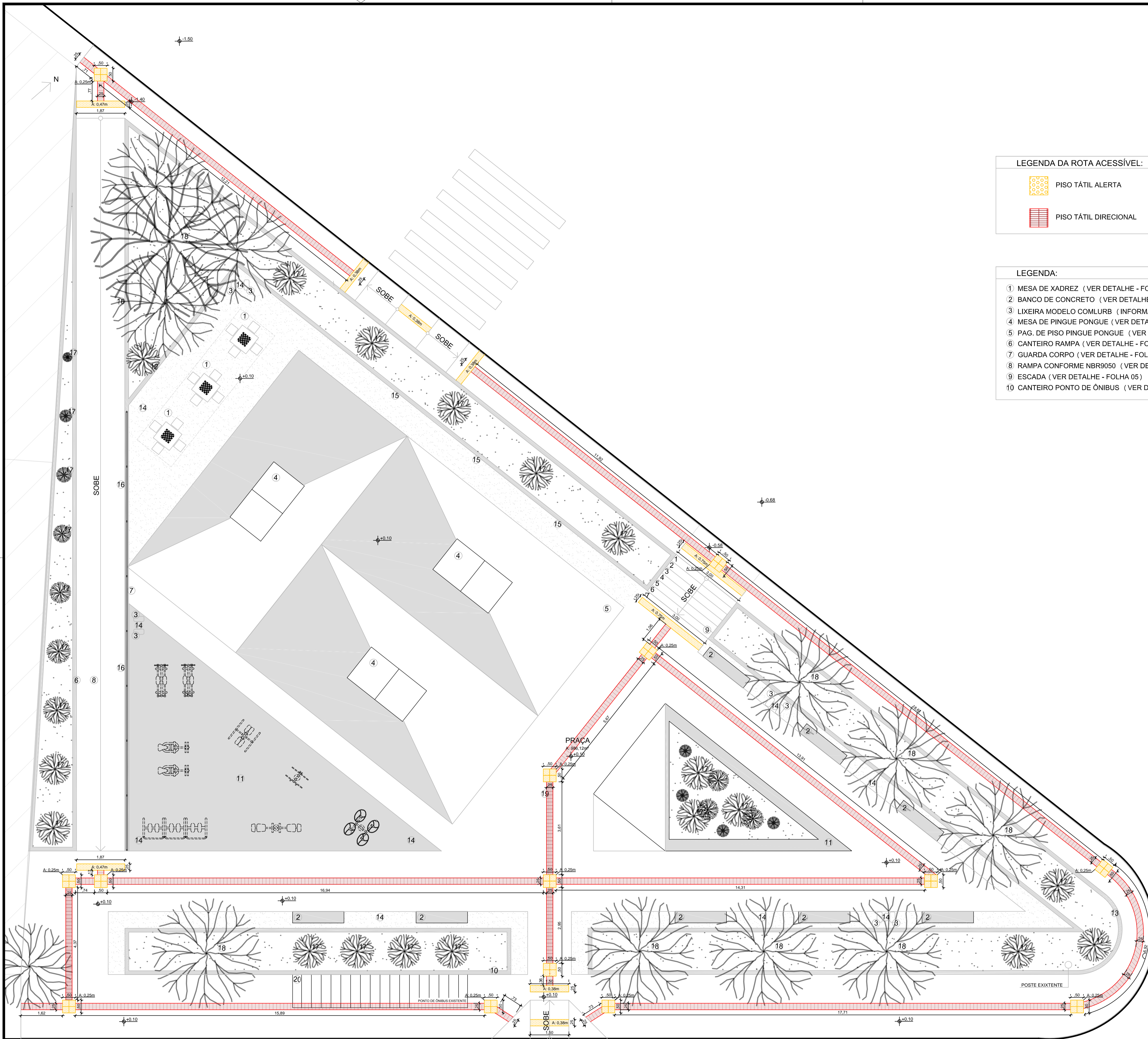
PLANTA BAIXA - ROTA ACESSÍVEL ESCALA 1:75
