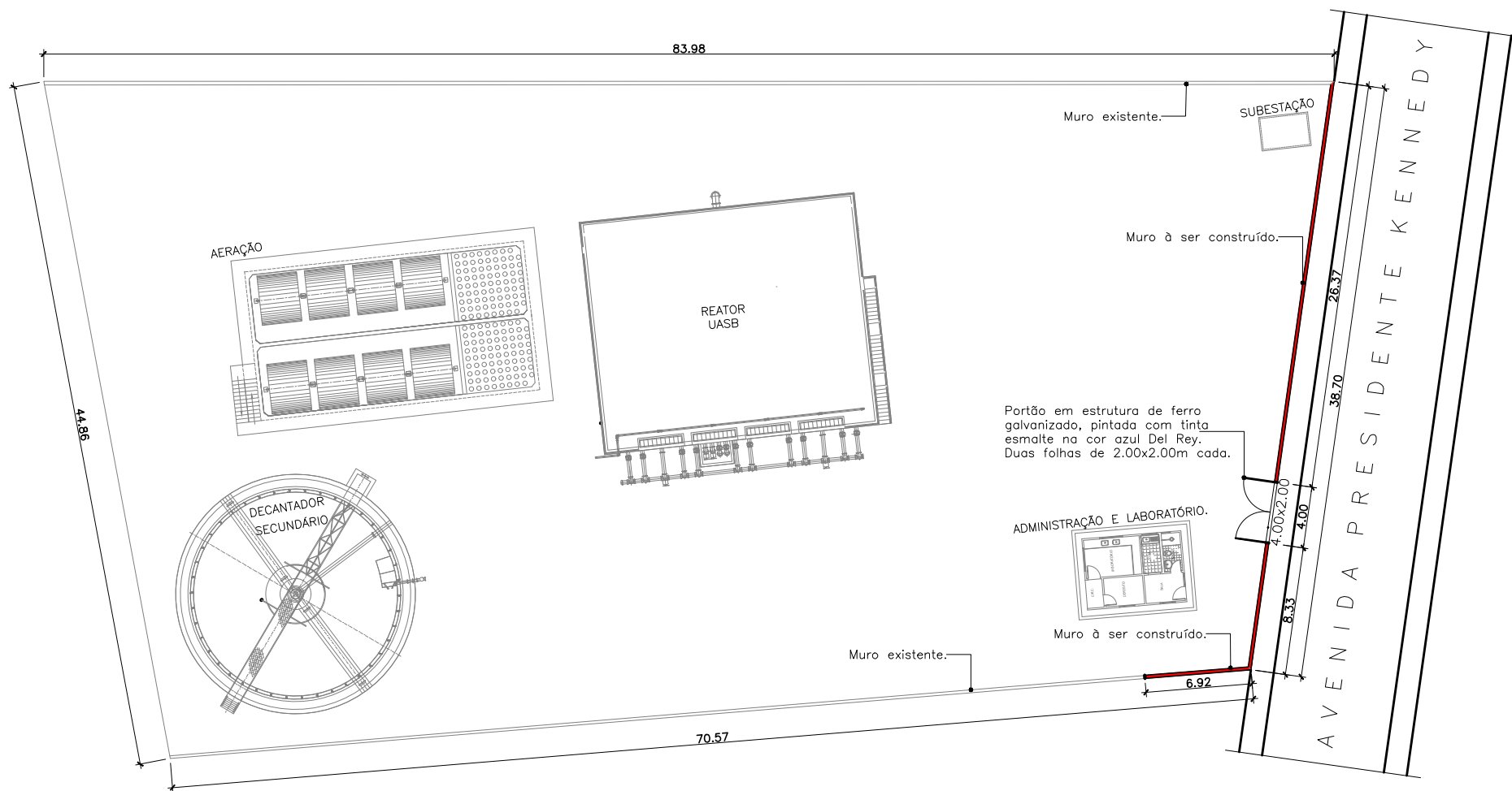
PLANTA À CONSTRUIR ESC.: 1:400
